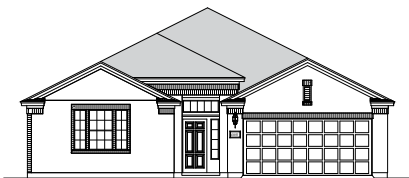
ELEVATION A
